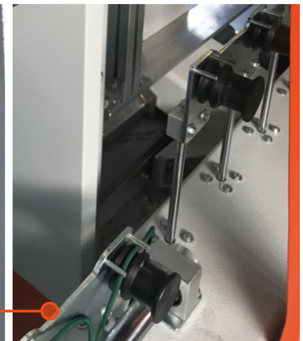
Sistema di appoggio vetro composto da rulli motorizzati montati su cilindri pneumatici che consentono la scomparsa del rullo in caso di lavorazione
