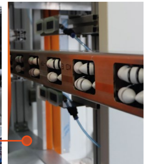
Barra di appoggio verticale mobile composta da rotelle omni-direzionali in materiale antigraffio
