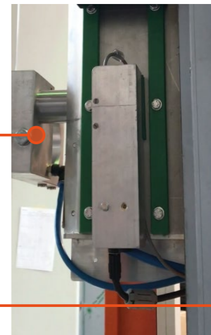
Sensore di rilevazione zero pezzo montato direttamente sull'unità operatrice
