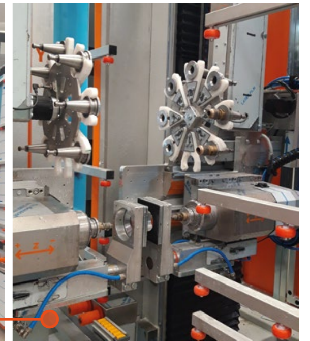
Magazzino utensili a 8/10 posizioni che permette un cambio utensile molto rapido
