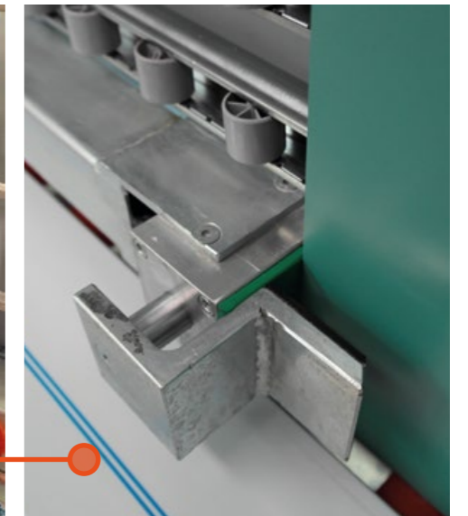
Pinza di bloccaggio e trasporto del vetro
