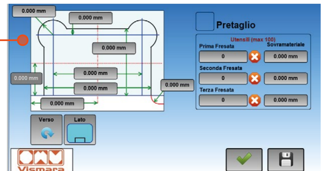
Interfaccia operatore di facile uso e comprensione con libreria di figure parametriche impostabili
