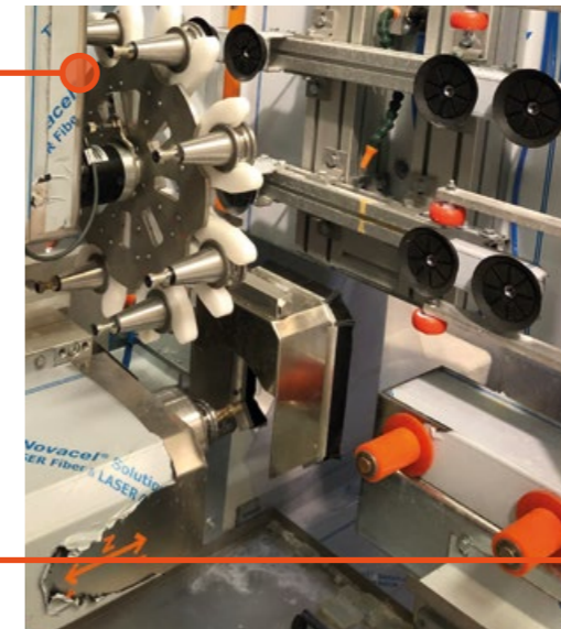
Ventose di bloccaggio e movimentazione vetro durante lavorazione di fresatura
